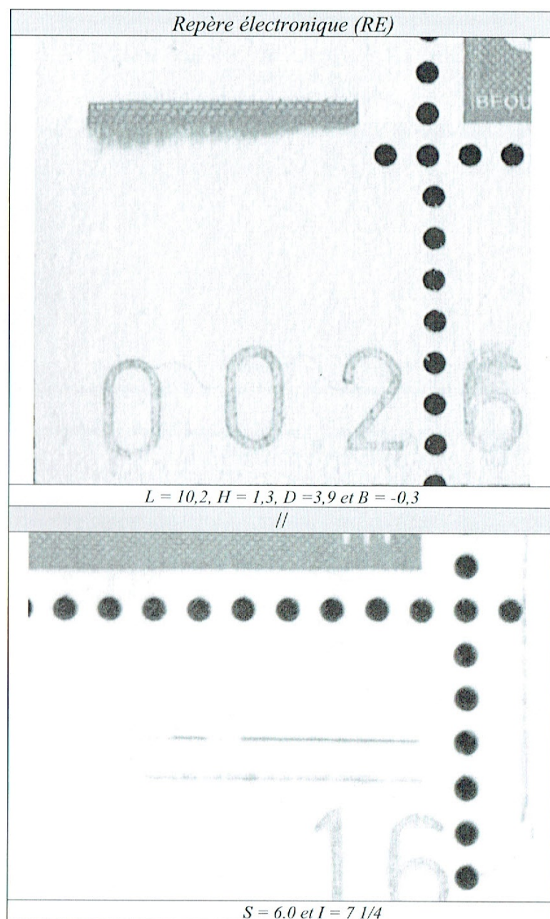
Figure 1 : Caractéristiques du cylindre AM
